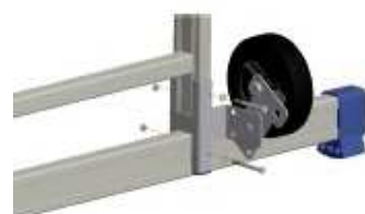
Bezpečnostní pozice koleček v případě použití rámu jako samostatného žebříku.
